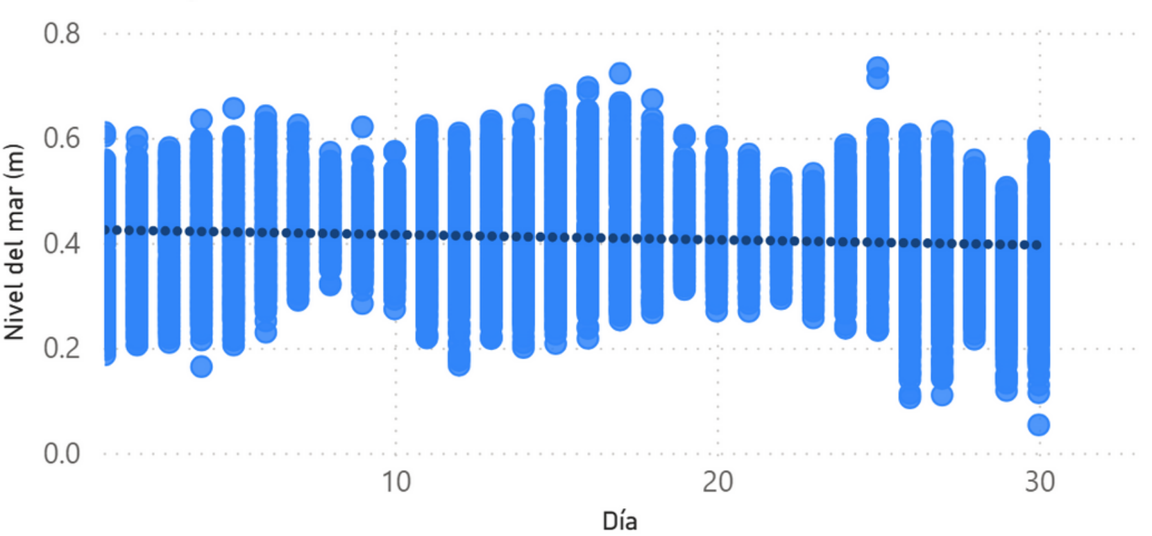
Nivel del mar en la costa sur de la República Dominicana para el mes de septiembre, 2025.
