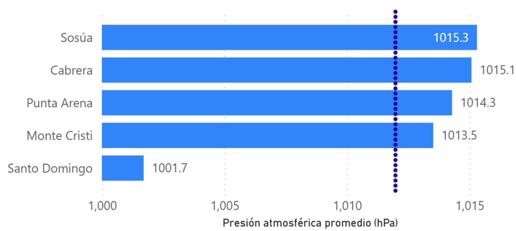
Presión atmosférica promedio por boya para el mes de septiembre, 2025.
