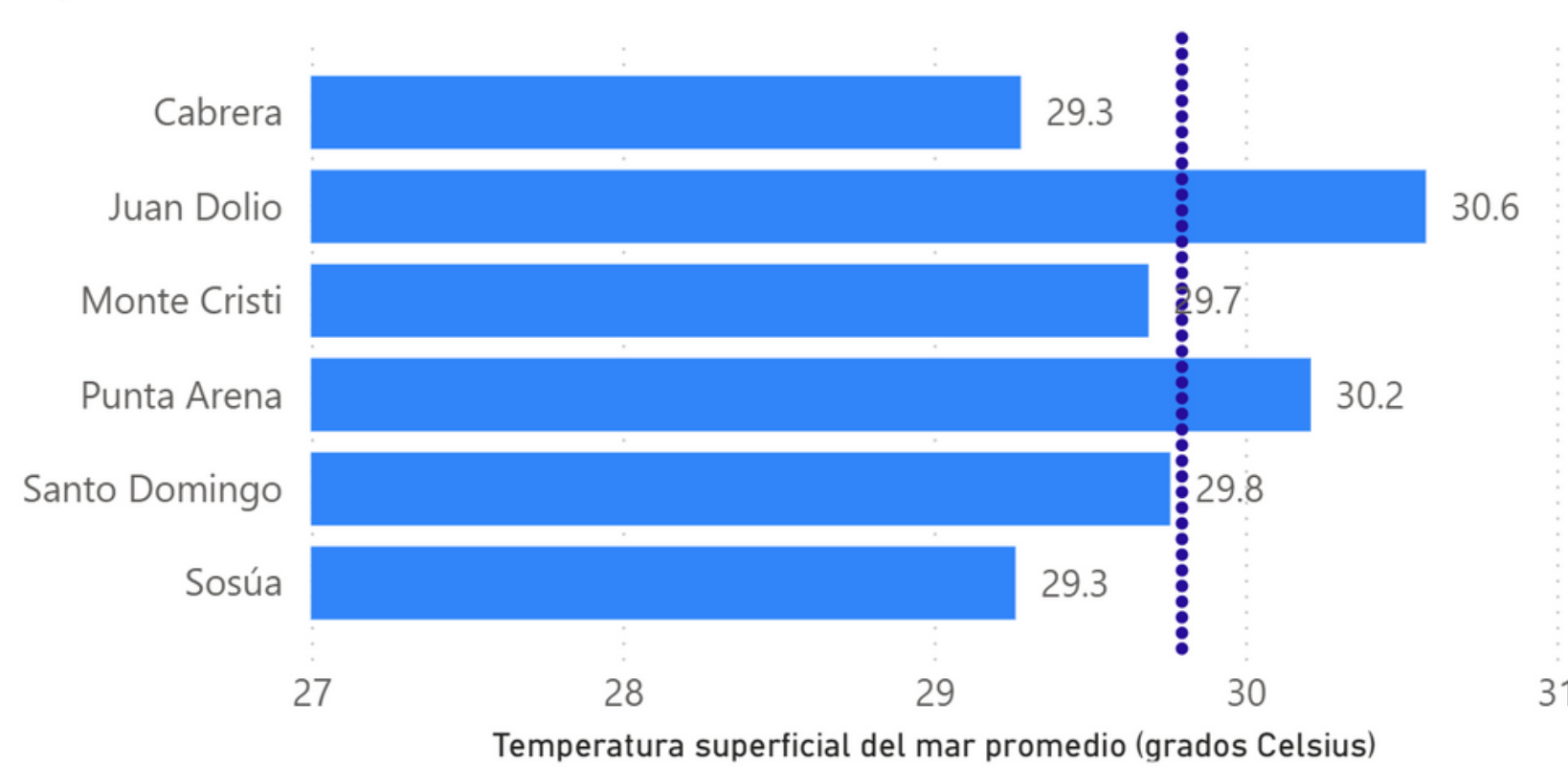
Temperatura superficial del mar promedio por boya para el mes de septiembre, 2025.
