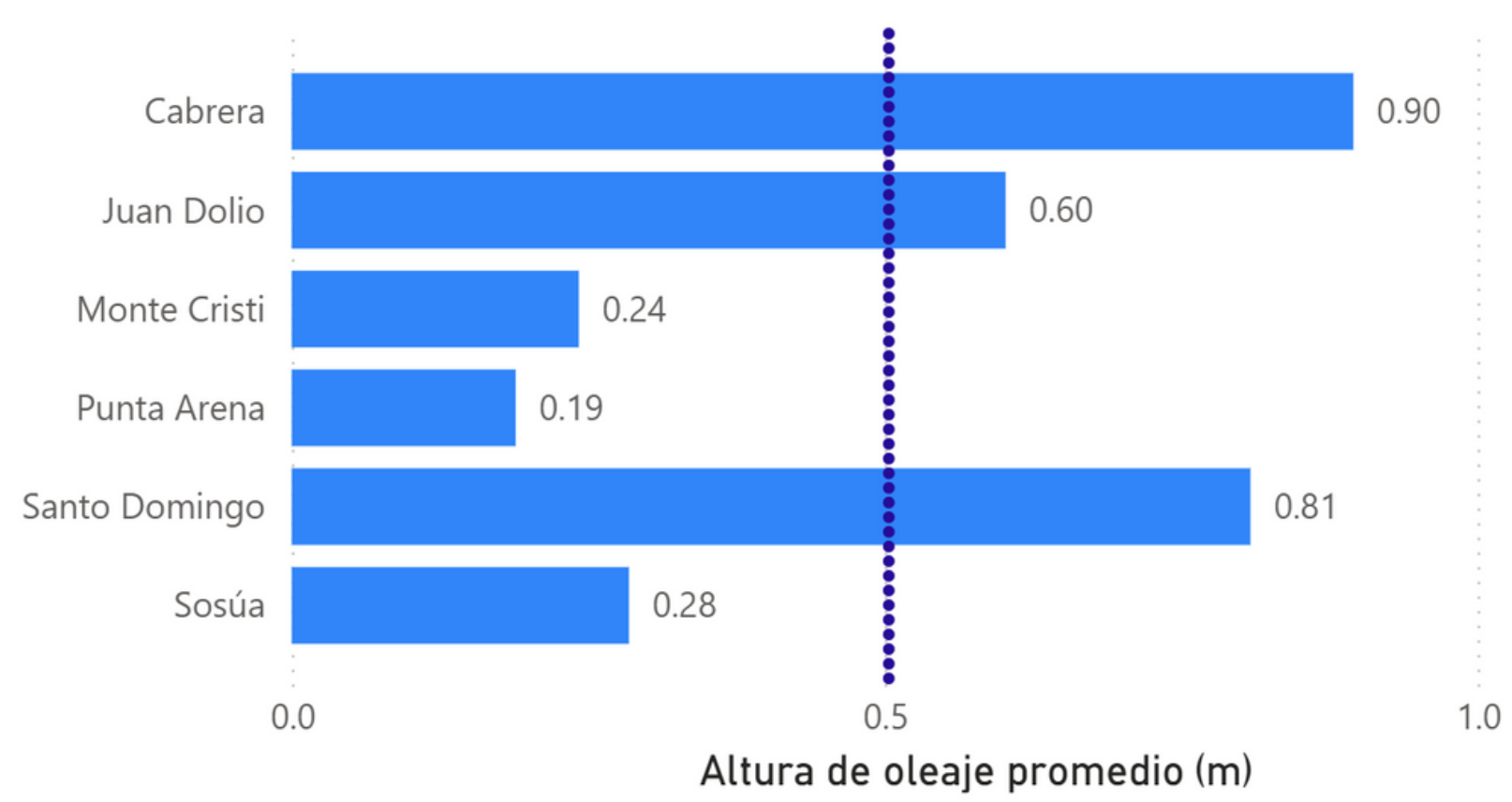
Altura de oleaje promedio por boya para el mes de septiembre, 2025.
