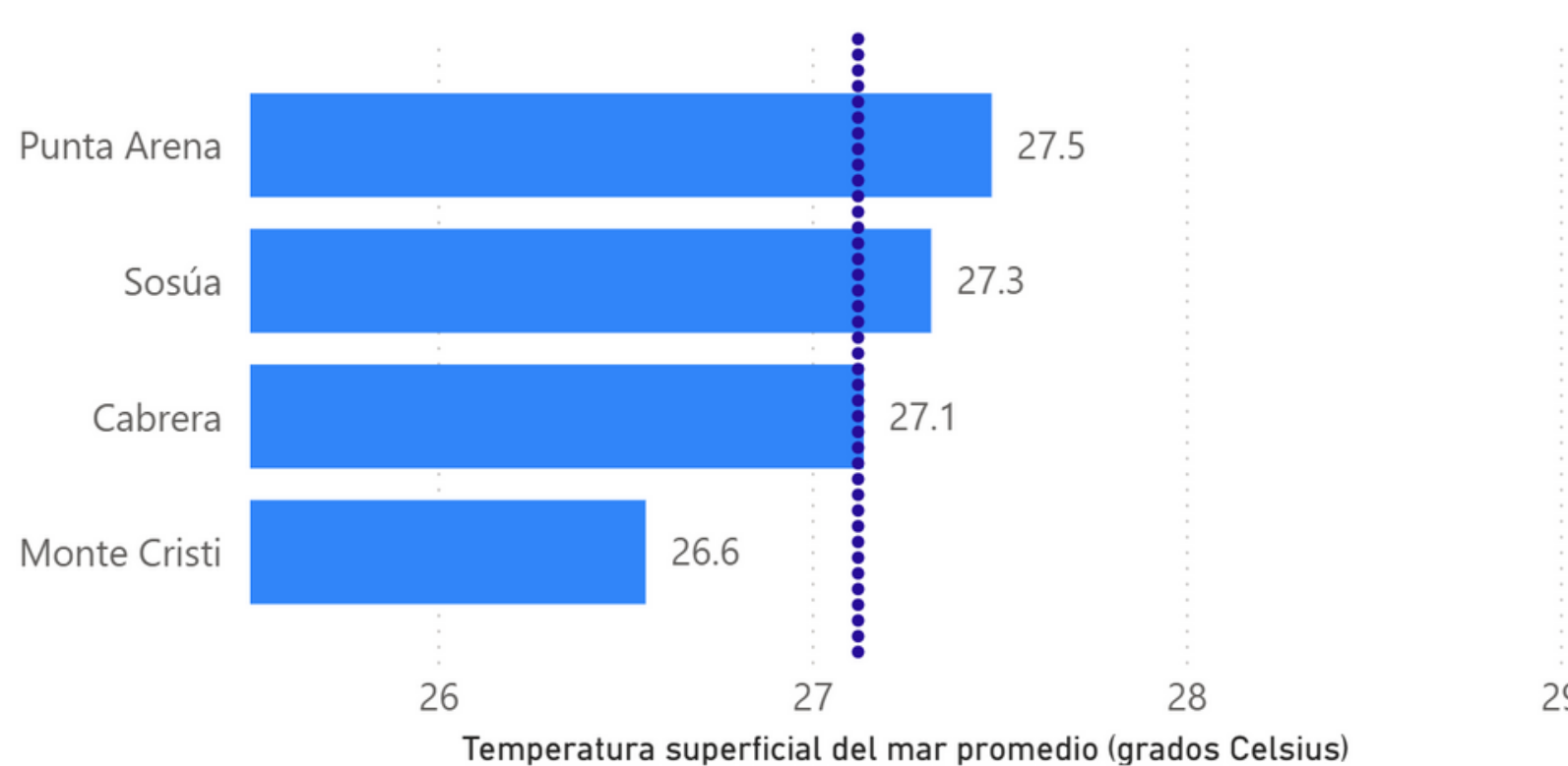
Temperatura superficial del mar promedio por boya para el mes de enero, 2026.
