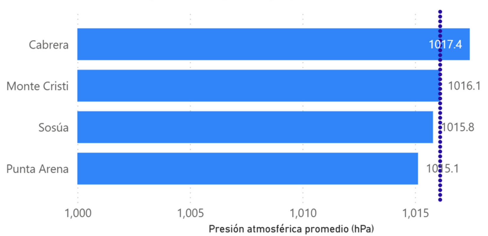
Presión atmosférica promedio por boya para el mes de enero, 2026.
