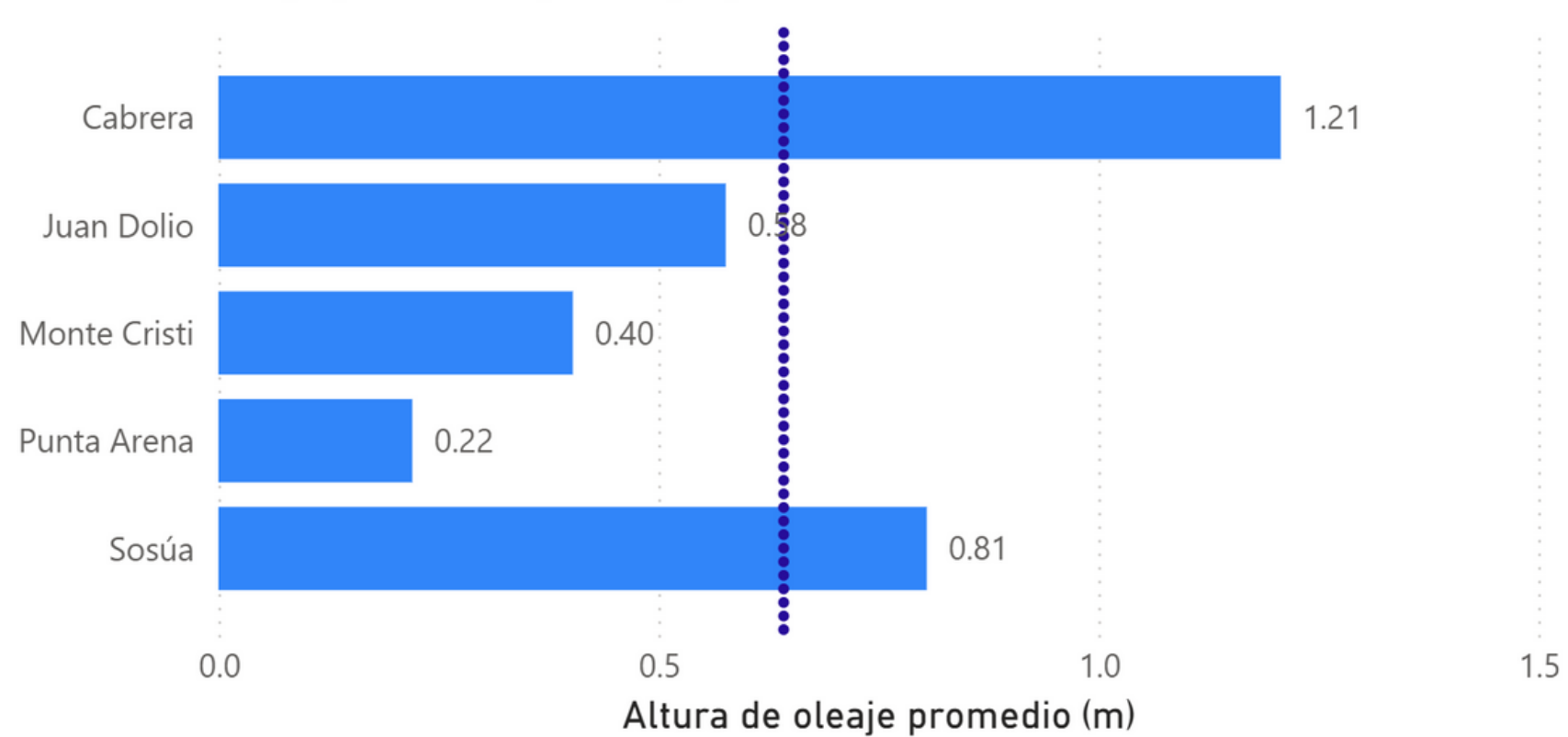
Altura de oleaje promedio por boya para el mes de enero, 2026.
