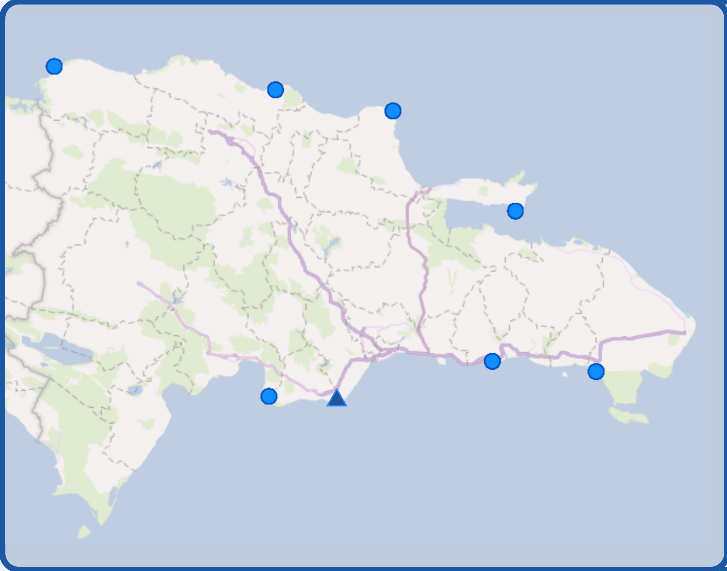
Altura de oleaje promedio por boya para el mes de enero, 2026.
