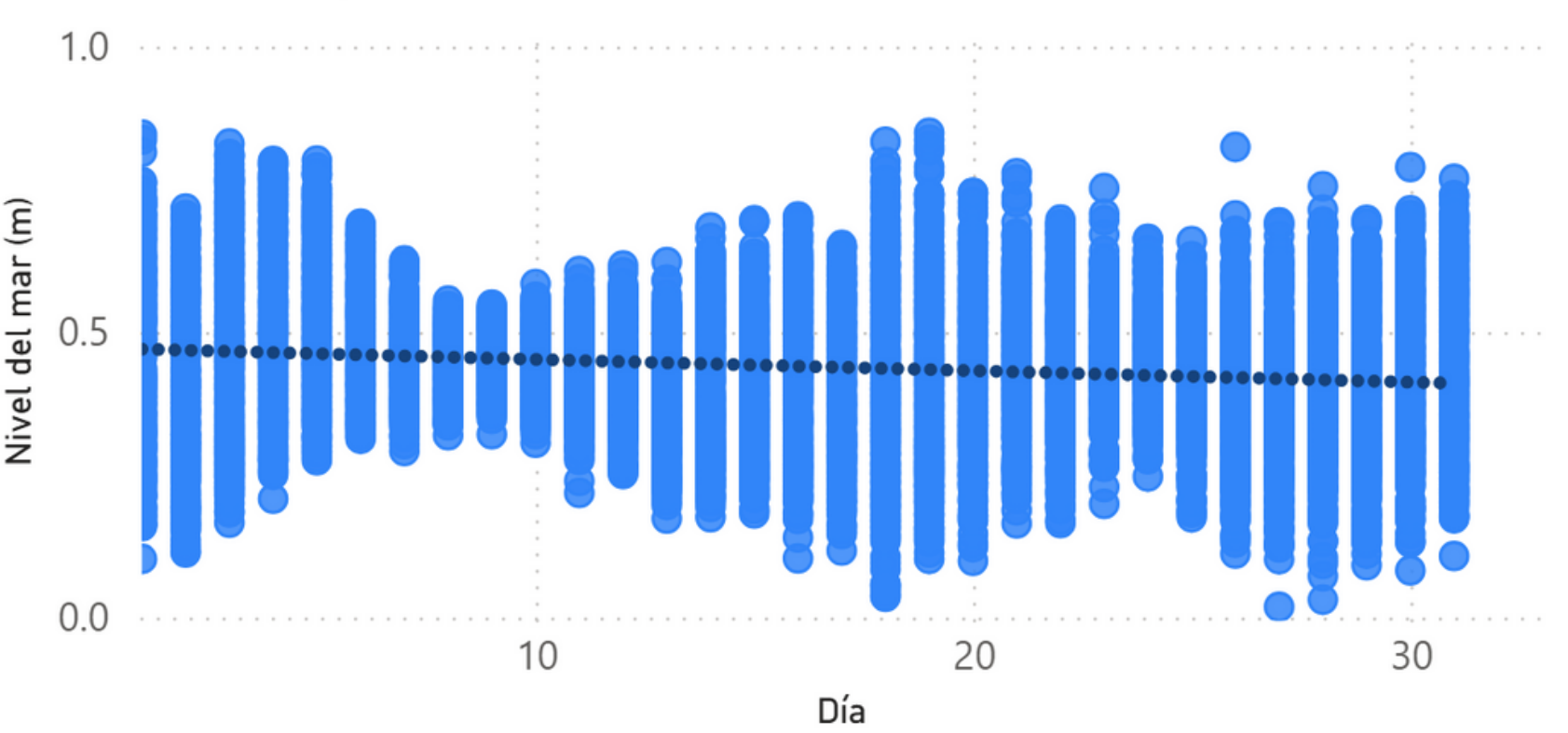
Nivel del mar en la costa sur de la República Dominicana para el mes de enero, 2026.
